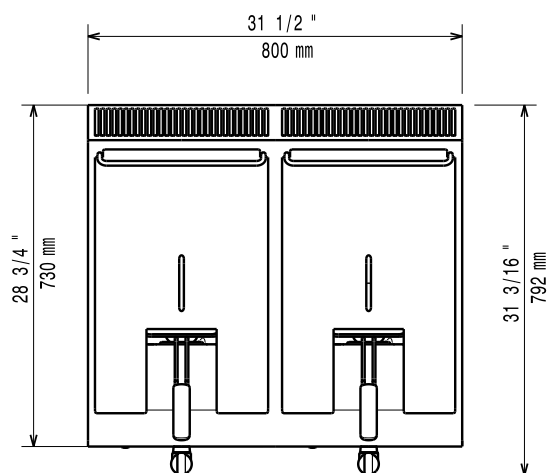
Felülnézet
